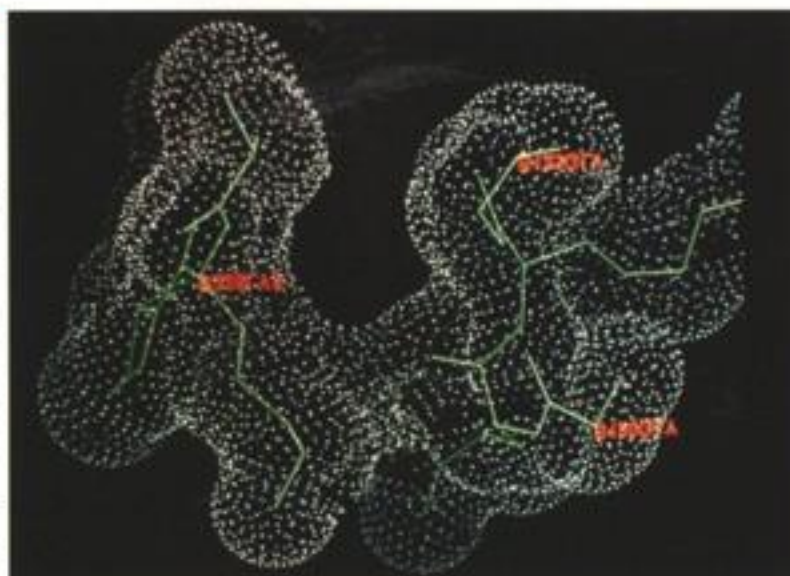
ТАК ВЫГЛЯДИТ МОЛЕКУЛА СИНТЕТИЧЕСКОГО ГОРМОНА «ХУМАЛОГ» — НОВИНКИ ФИРМЫ ELI LILLY, ОТЛИЧАЮЩЕЙСЯ ОТ НАТУРАЛЬНОГО ИНСУЛИНА ДВУМЯ АМИНОКИСЛОТАМИ И БОЛЕЕ БЫСТРЫМ ДЕЙСТВИЕМ
